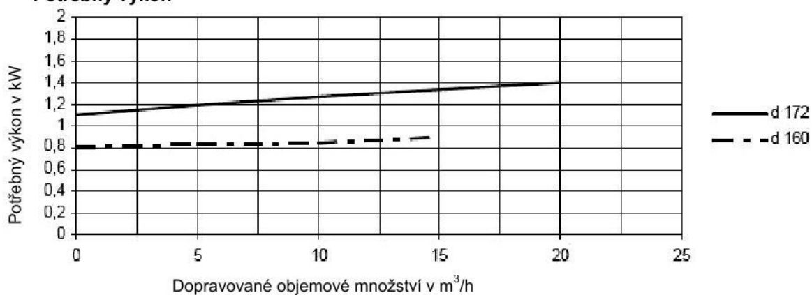
Potřebný výkon
