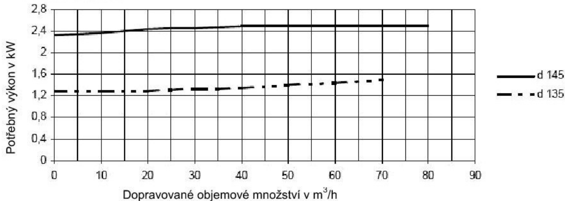
Potřebný výkon
