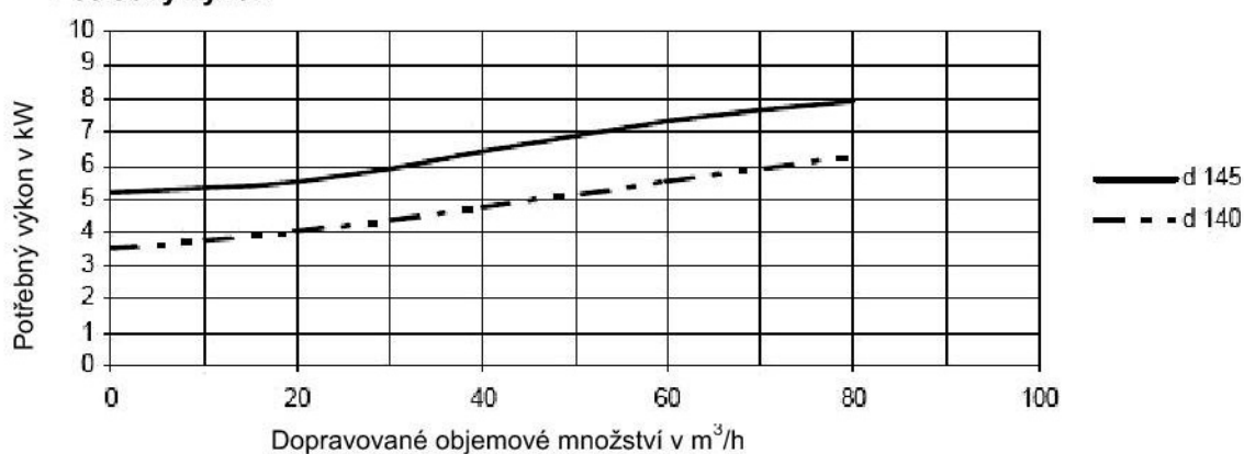
Potřebný výkon
